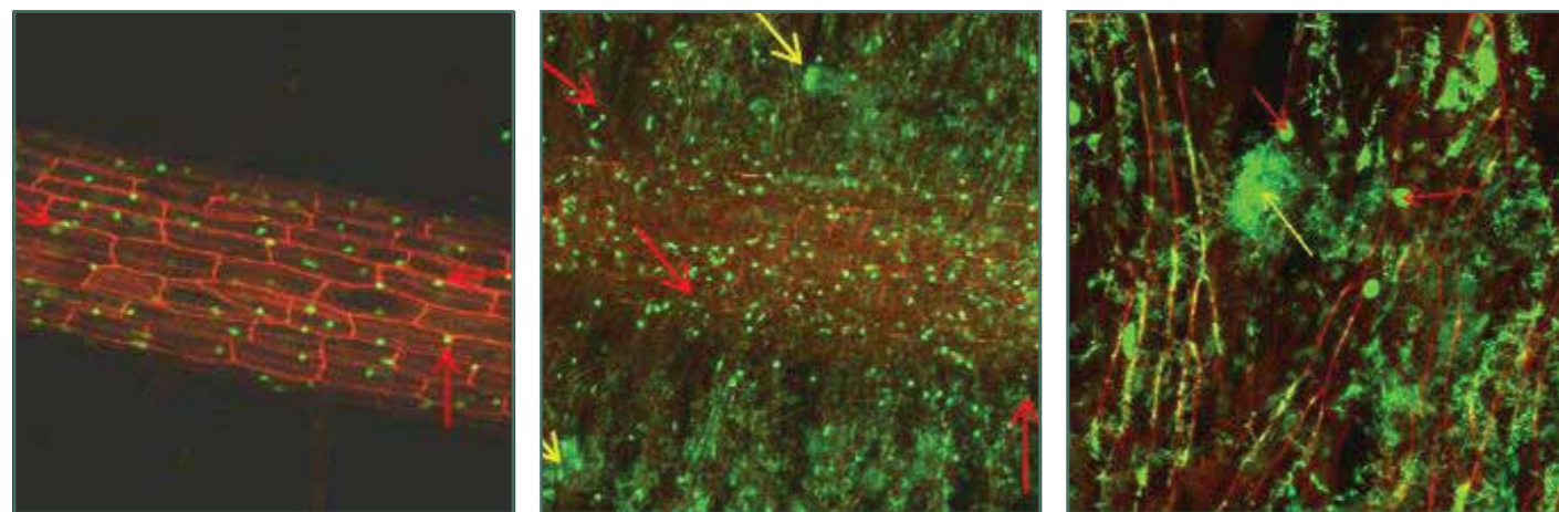
Kezeletlen paradicsomgyökér
