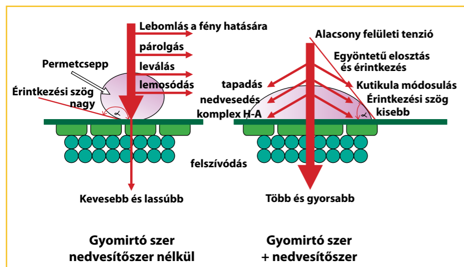
Nedvesítőszer hatásmódja
